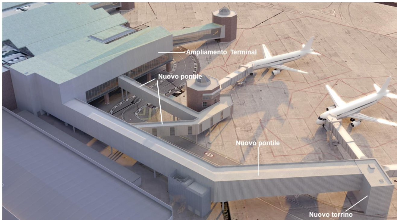
Viste 3D esterna dell'ampliamento Pier Sud e dei diversi elementi architettonici (ampliamento terminal, pontili di imbarco/sbarco, torrino. I finger, visibili nelle immagini, sono esclusi dal presente appalto)
