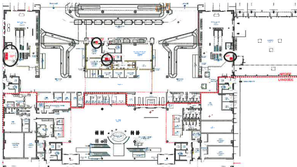
Aerostazione piano terra
